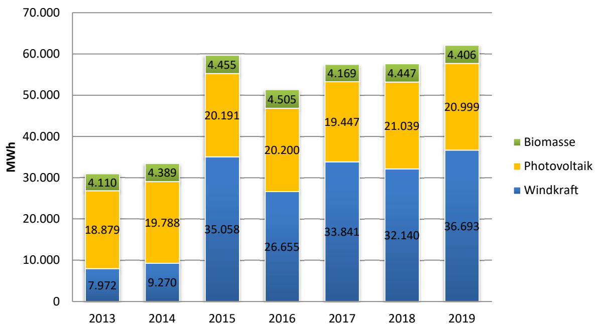
Abbildung 13: Stromerzeugung durch Erneuerbare Energien in Wolfhagen
